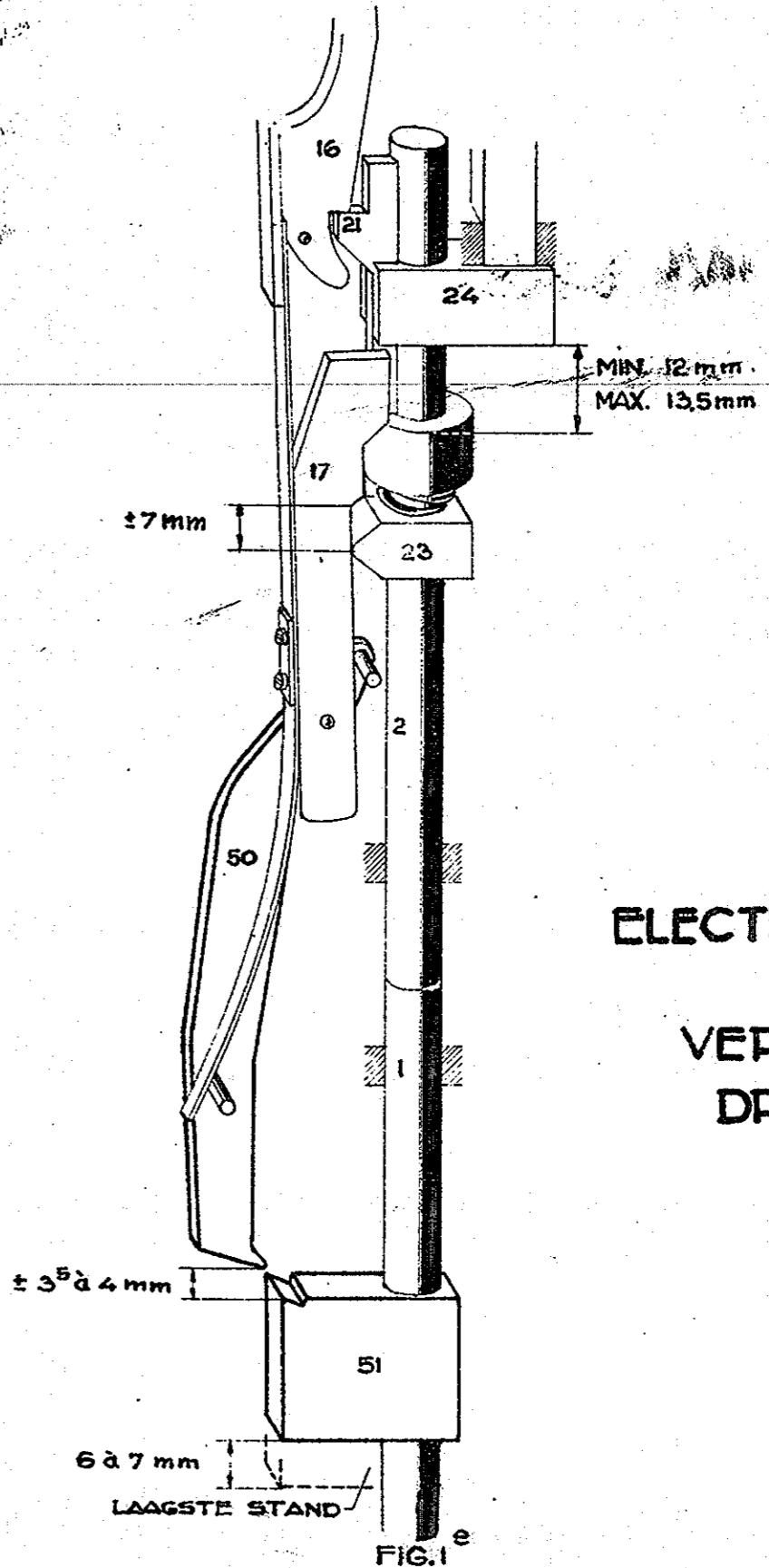
FIG. 1 e BLOKKNOP LOSGELATEN NA STROOMGAVE. BOVENSLUITPEN BLUFT IN GEDRUKTE STAND STAAN; DAARDOOR OOK DE ONDERSLUITPEN. PAL 17 IS NAAR RECHTS BEWOGEN (ONDER 24), DAARDOOR VOET VAN PAL 50 NAAR LINKS.
