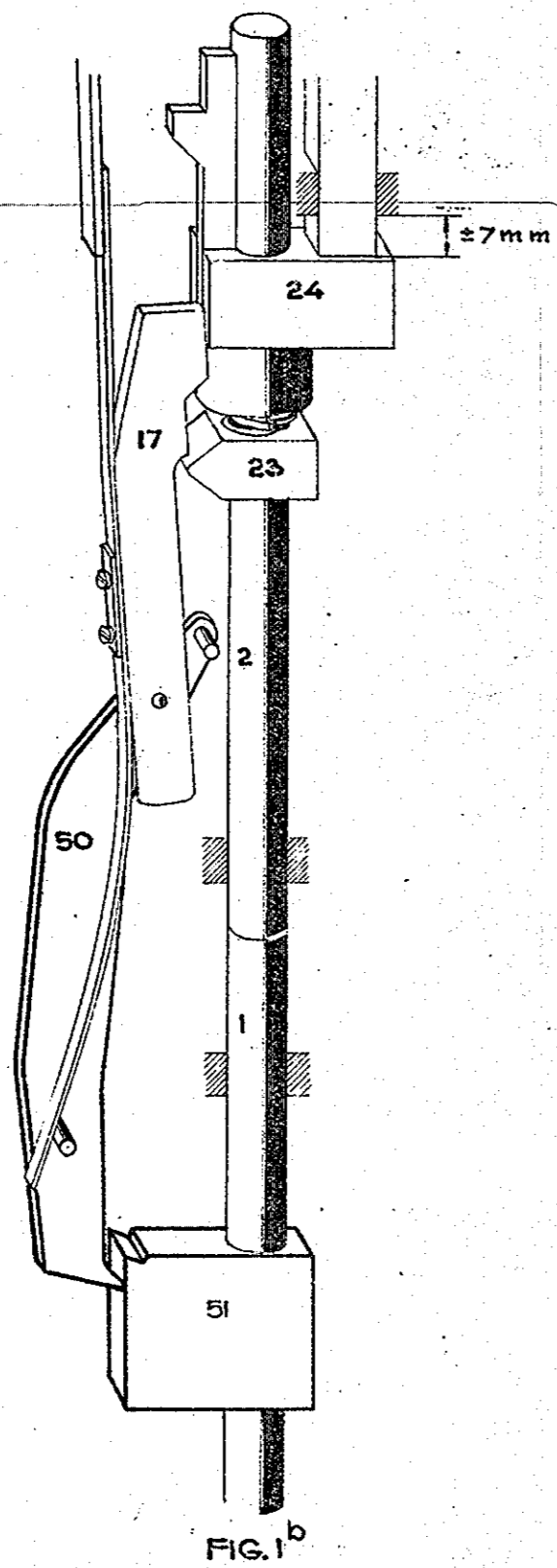
FIG. 1 b SLOT ZOVER GEDRUKT, DAT STUITING VAN PAL 17 DOOR NOK 23 OVERGENOMEN IS DOOR DWARSSTUK 24.
