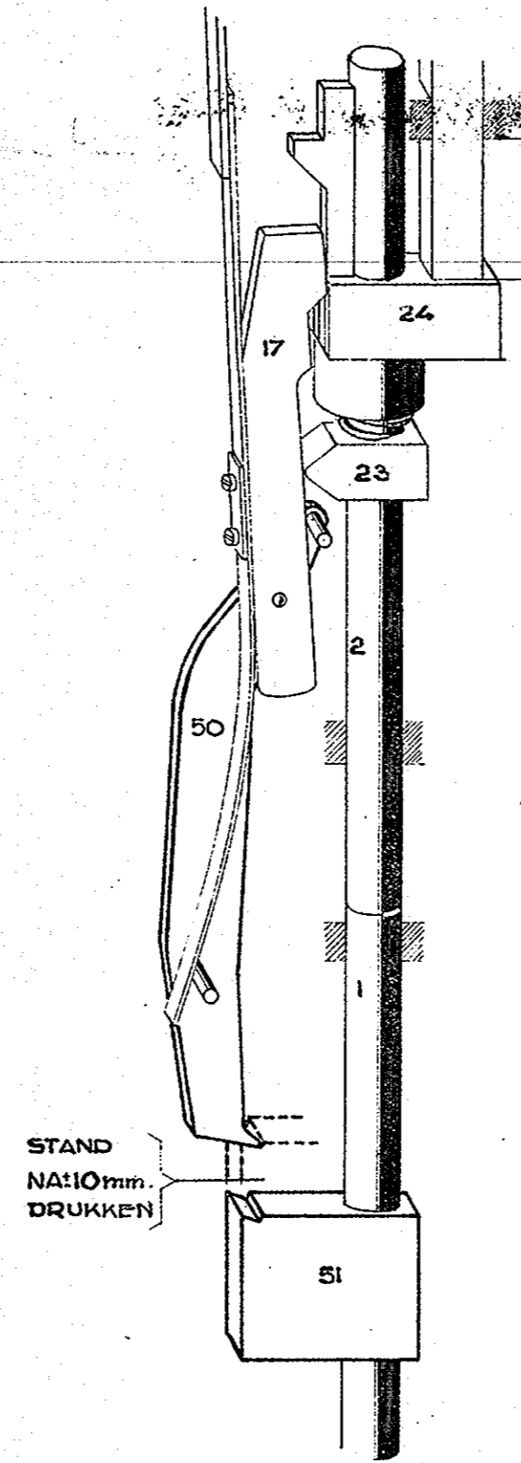
FIG. 1 c SLOT GEHEEL GEDRUKT; PAL 50 IS VRUGEKOMEN VAN NOK 51, EN DE VOET IS NAAR RECHTS BEWOGEN.
