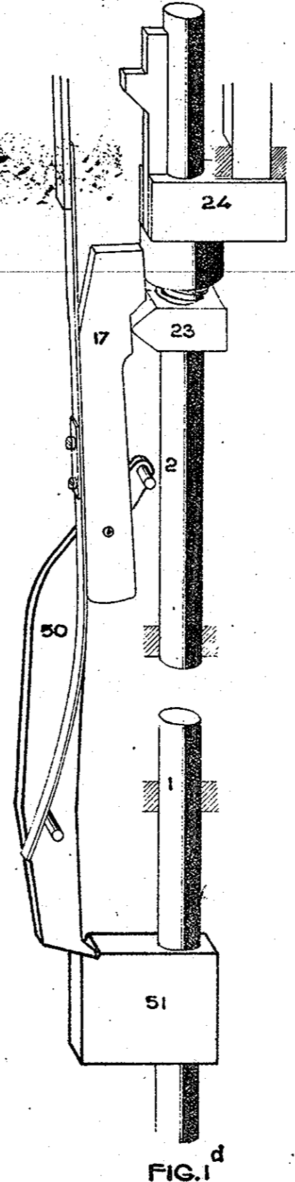
FIG. 1 d BLOKKNOP LOSGELATEN; STROOMGAVE VOND NIET PLAATS. PAL 17 BLUFT NAAR LINKS GEDRUKT; NOK 51 STUIT TEGEN PAL 50 (PAL VOOR VOLLEDIG BLOKKEN NIET AANWEZIG GEDACHT).
