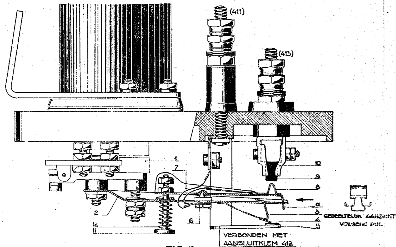
FIG. 2 DOORSNEDE VOLGENS A-B, FIG. 3
